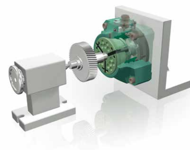
Bearbeitung von langen Teilen, beispielsweise mithilfe eines Reitstocks zur Abstützung.
