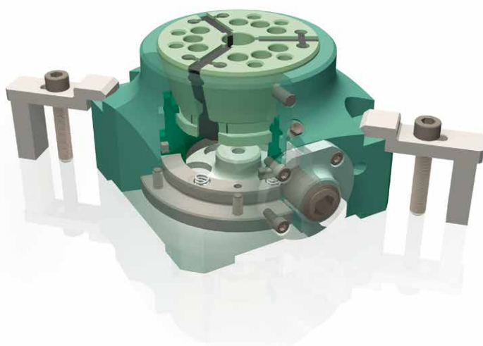
Befestigung durch direkte Verschraubung auf dem Montagetisch mit oder ohne Pratzenspannung.
