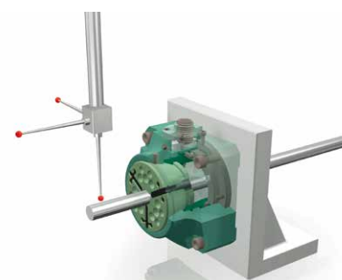
Befestigung an Winkelplatte – auch mit Durchlass – für die ein- oder zweiseitige Bearbeitung.
